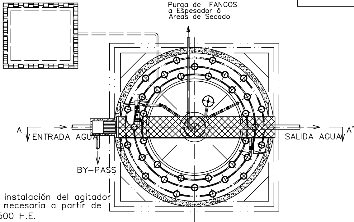
PLANTA
