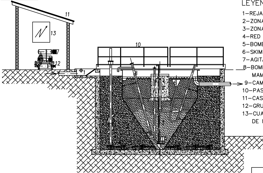
CORTE A-A'
